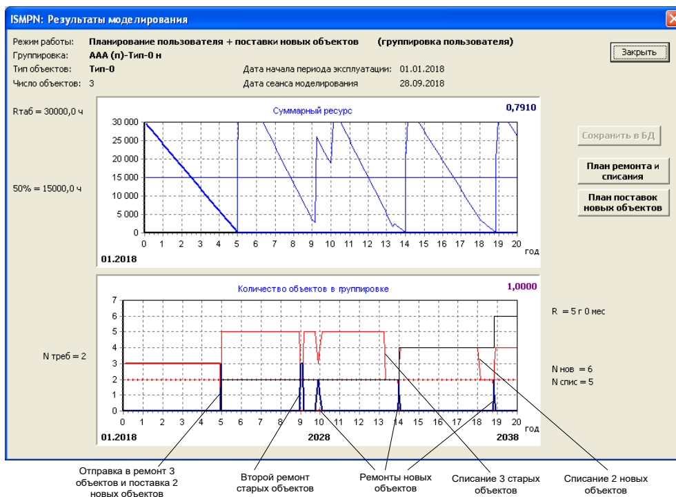
Рисунок 7 – Результати моделювання в режимі Нормативне планування + поставка новых об'єктів (угруповання користувача, об'єкти Тип-0, тестові дані)
