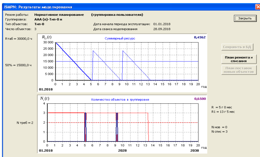
Рисунок 5 – Результаты моделирования в режиме Нормативне планування (Угруповання користувача, об'єкти Тип-0 , тестові дані)
