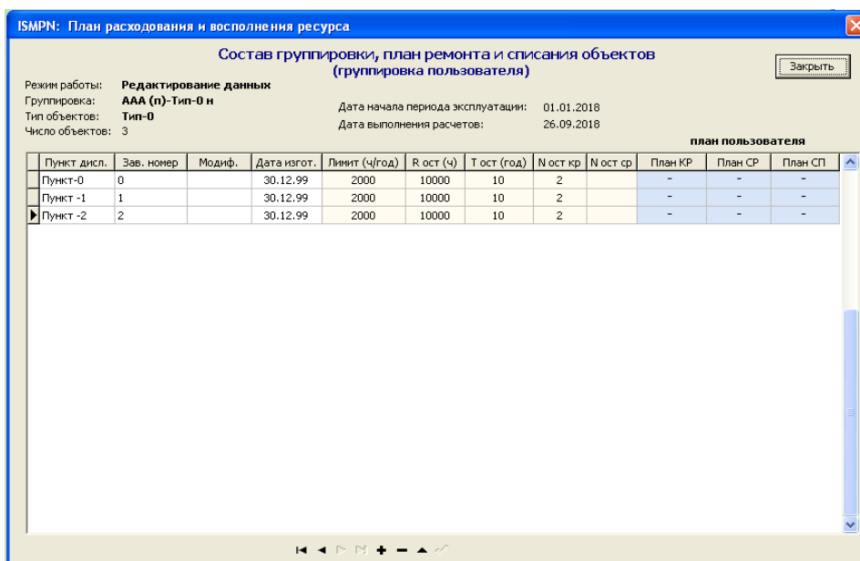
Рисунок 4 – Вигляд екрану ПК в режимі редагування угруповання користувача
