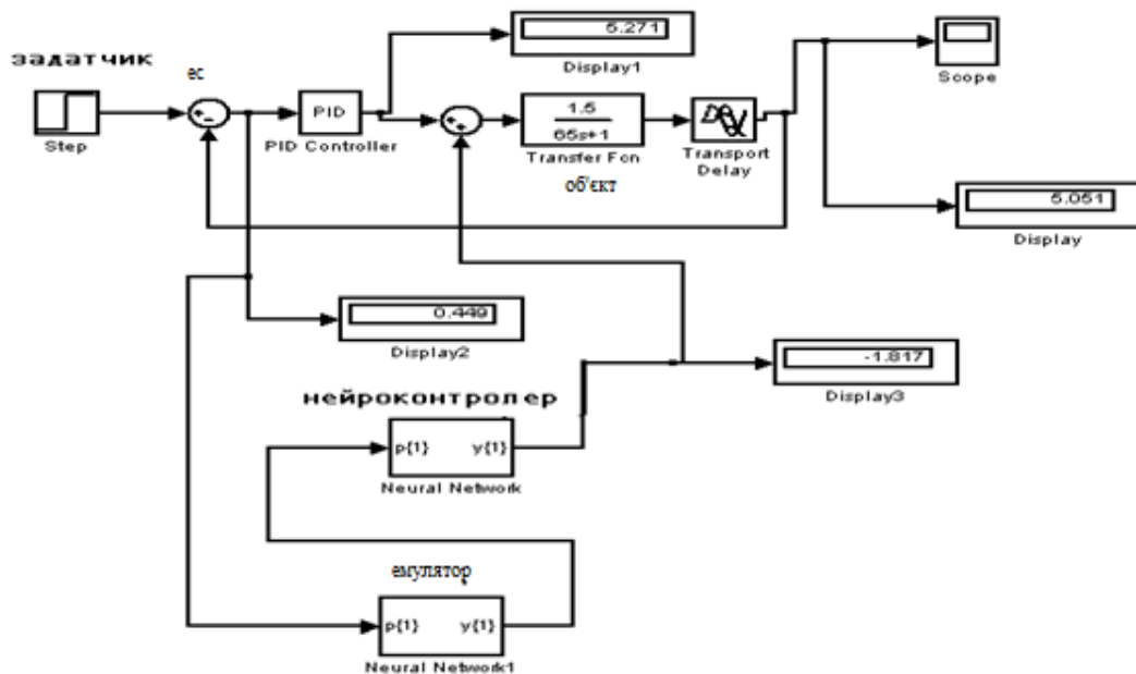
Рисунок 3. Схема нейромережевого управління (НМК) з емулятором та ПІД-регулятором
