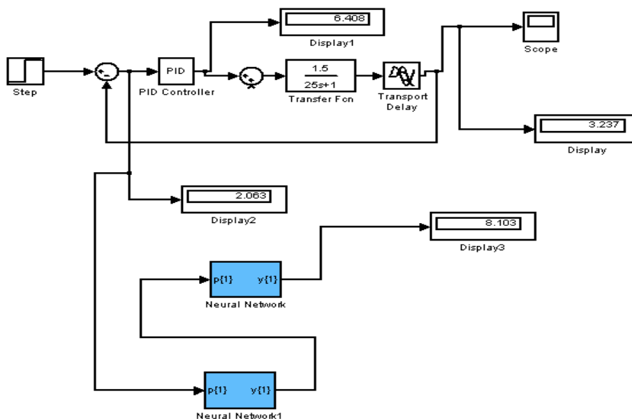
Рисунок 5. САУ з ПІД – регулятором при дії внутрішнього збурення
