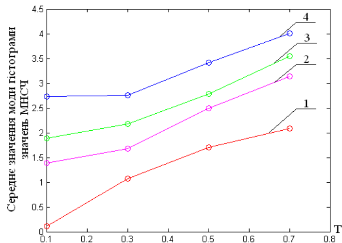
Рисунок 4. Графіки залежності середнього по експерименту значення моди гістограм значень елементів МНСЧ від параметру T : 1 – ЦЗ з множини Y ; 2, 3, 4 – відповідні ЦЗ з множин Y^{(80)} , Y^{(75)} , Y^{(70)} відповідно
