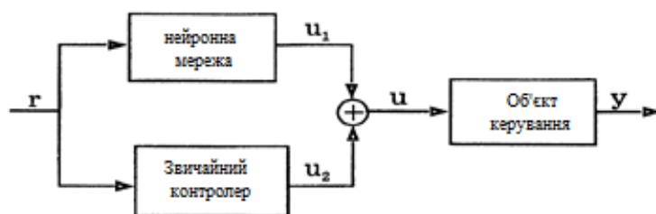
Рисунок 1. Паралельна схема нейроконтролера
