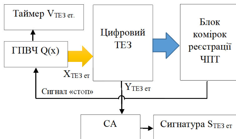
Рисунок 1. Структурна схема пристрою експериментальної будови тестової послідовності
