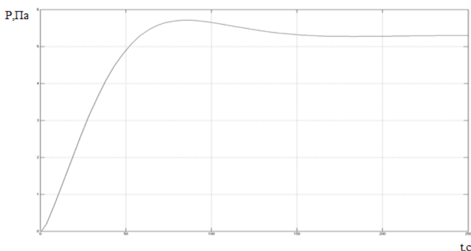
Рисунок 6. Перехідний процес ПІД - регулятора з об'єктом по каналу завдання
