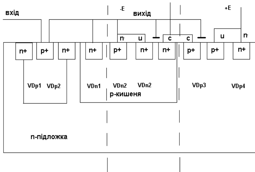
Рисунок 1 – Структурна великих інтегральних схем (BIC) і надвеликих інтегральних схем NBIC виготовлених за технологією “метал-діелектрик-напівпровідник”
