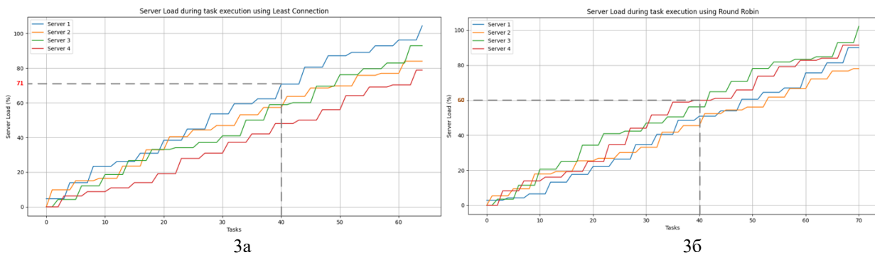
Рисунок 3 – Результати імітаційного моделювання отриманого розподілу ресурсів кластеру ( Round Robin , Least Connection )
