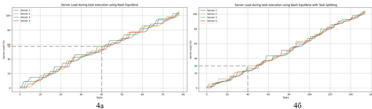
Рисунок 4 – Результати імітаційного моделювання отриманого розподілу ресурсів кластеру ( Nash Equilibria , Nash Equilibria with Task Splitting )
